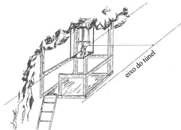
figura 3.42. Transferência de uma direcção num poço vertical
